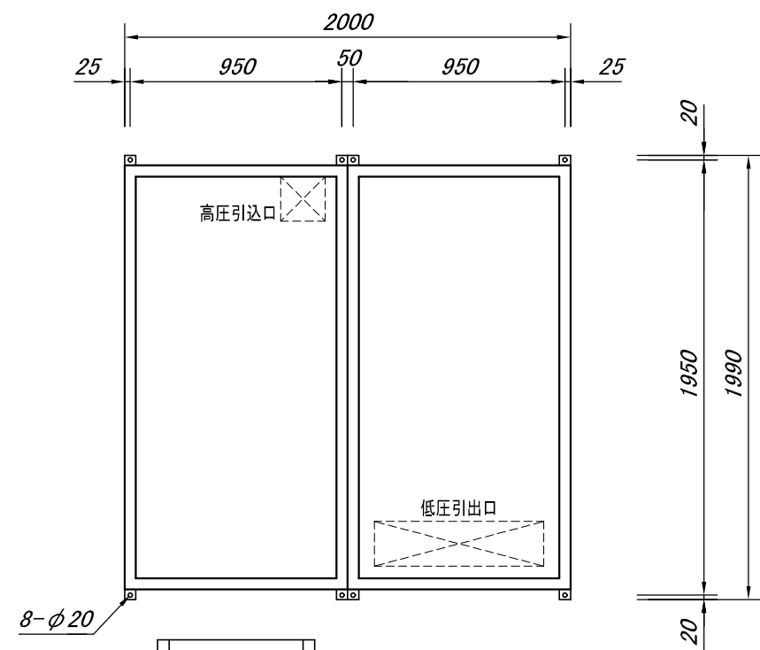
基礎図
