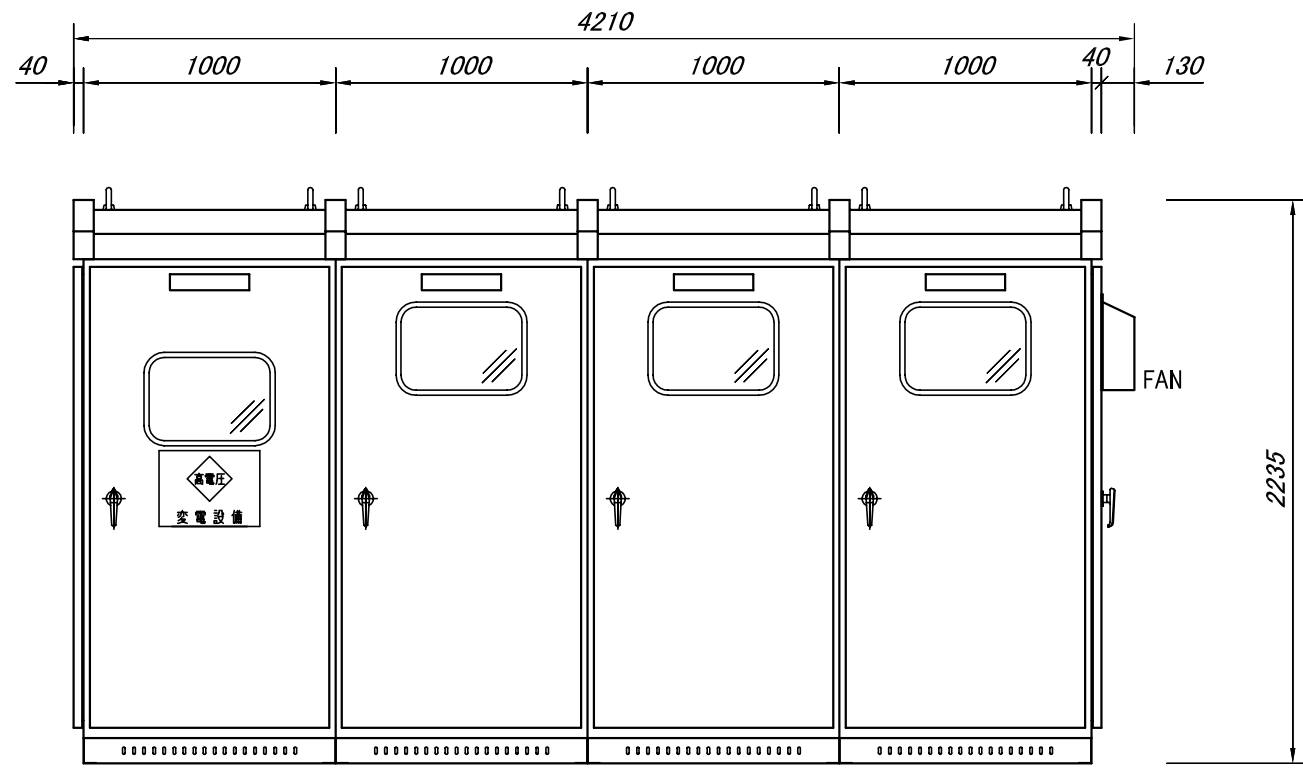
正面図
