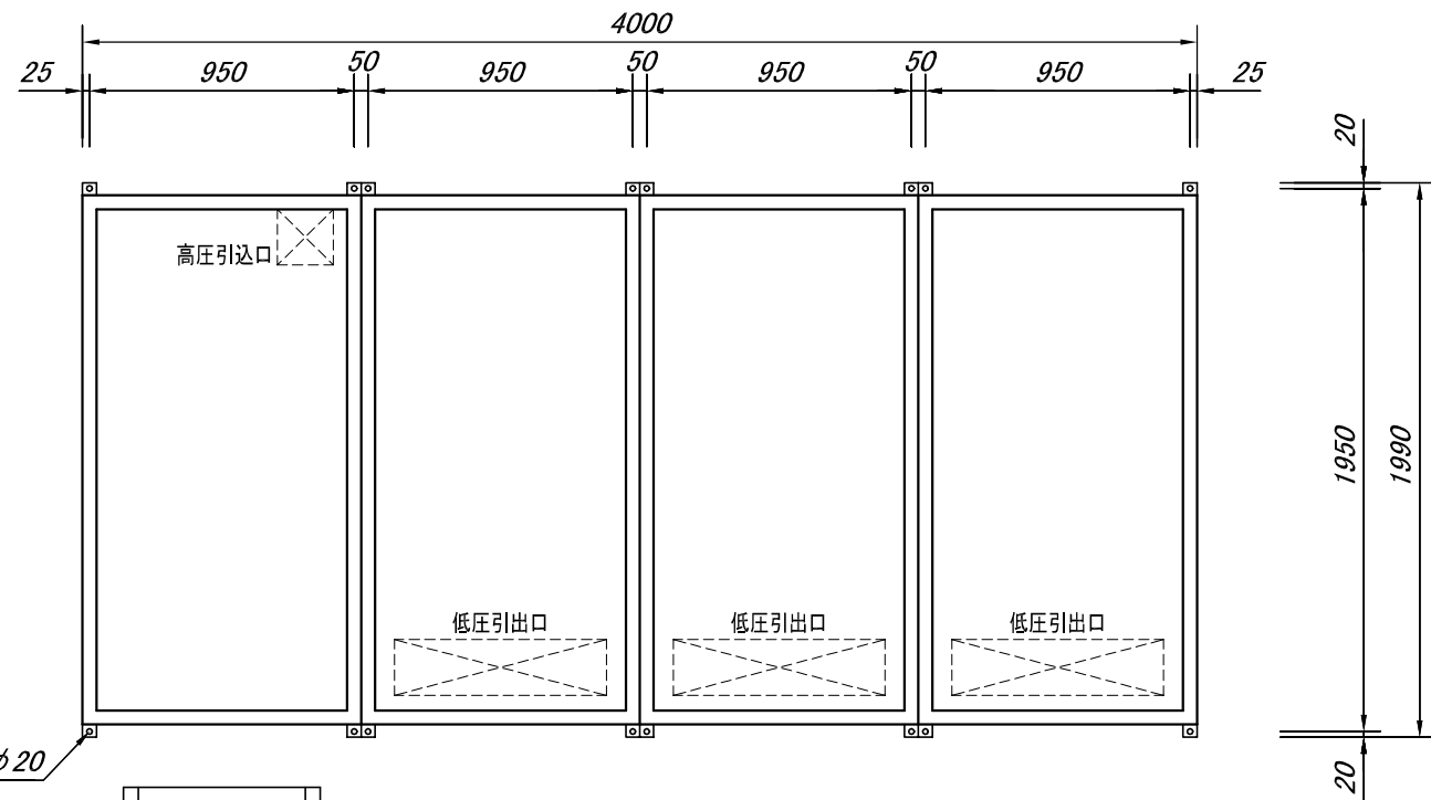
基礎図
